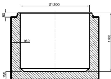
Espesor de pared y solera 160 mm
